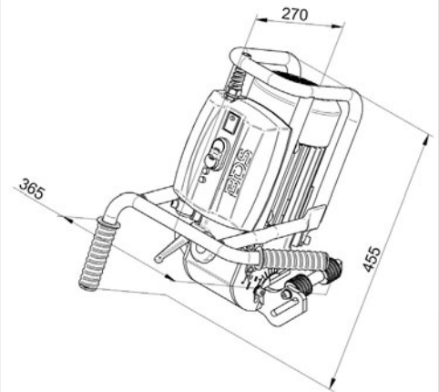
EKF 300, 450, 452
