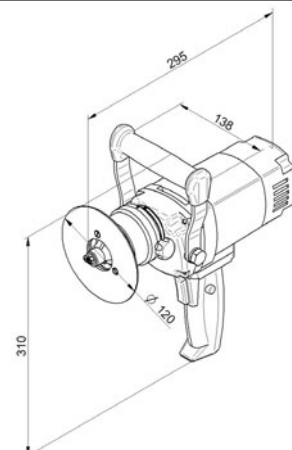
EKF 300, 450, 452
